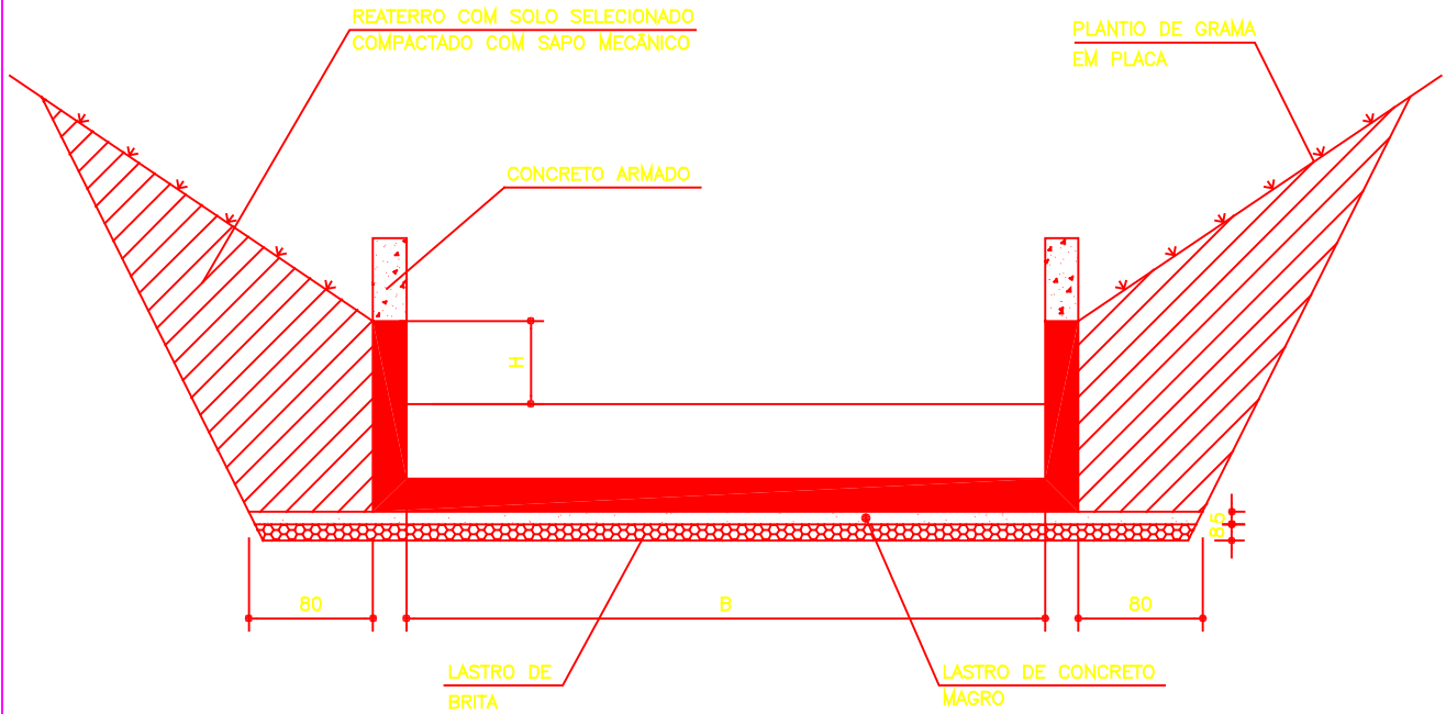
SEÇÃO TRANSVERSAL
