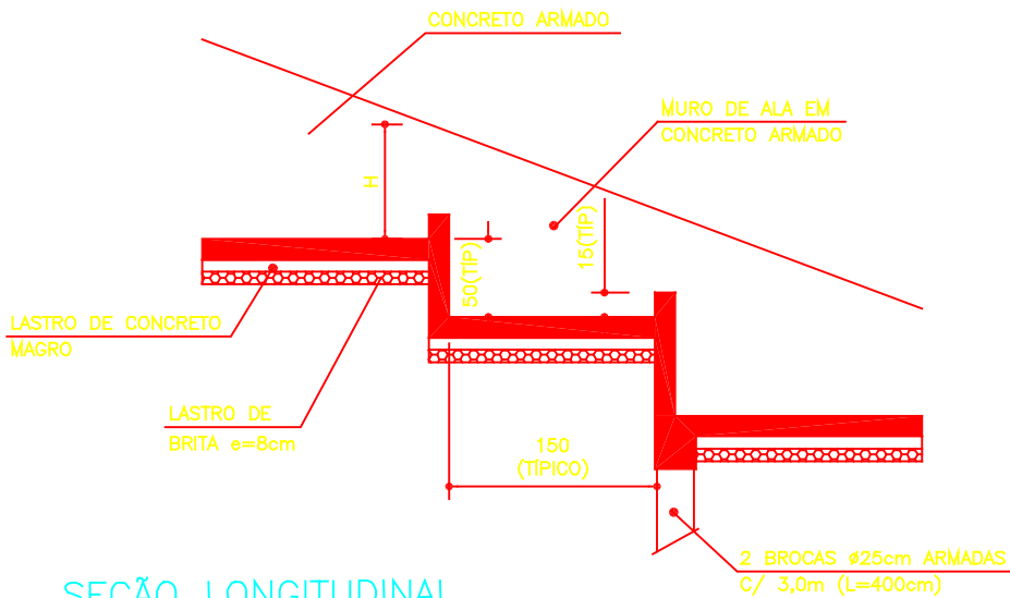
SEÇÃO LONGITUDINAL
