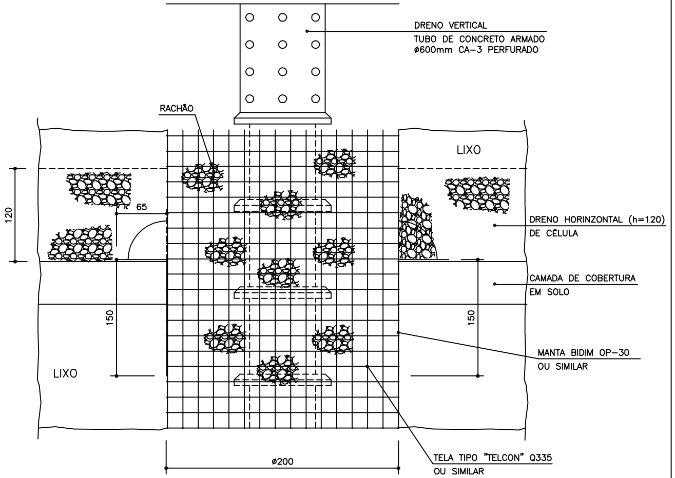
DETALHE TÍPICO JUNTO À COBERTURA DAS CÉLULAS
